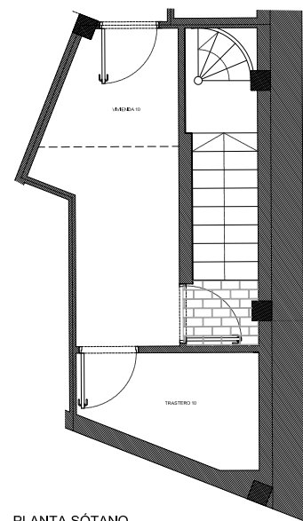
PLANTA SÓTANO
