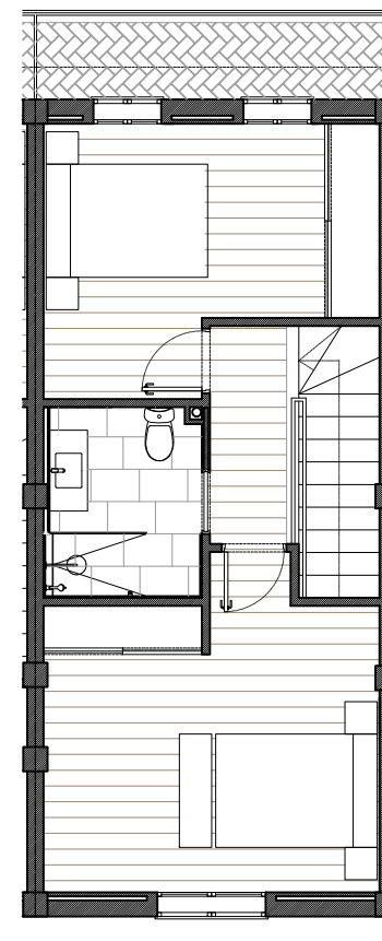
PLANTA PISO
