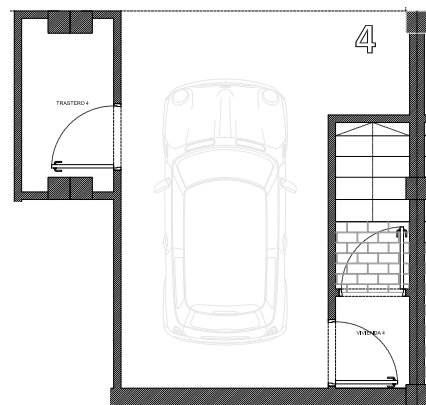
PLANTA SÓTANO
