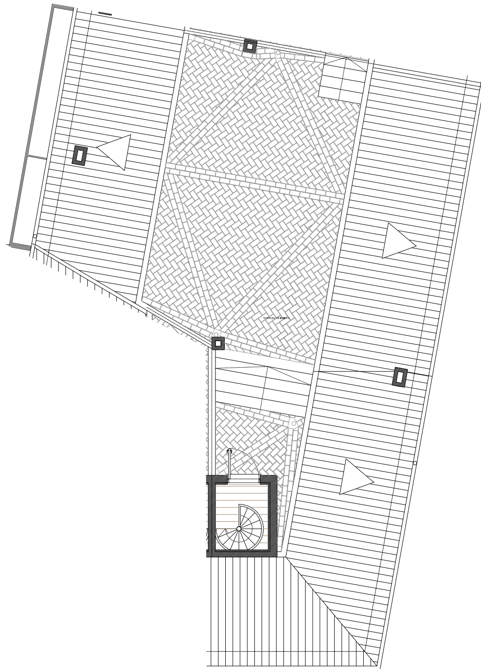
PLANTA AZOTEA
