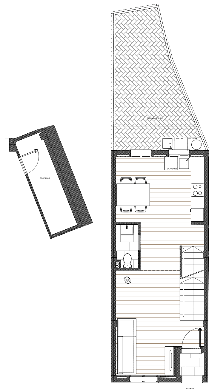
PLANTA BAJA
