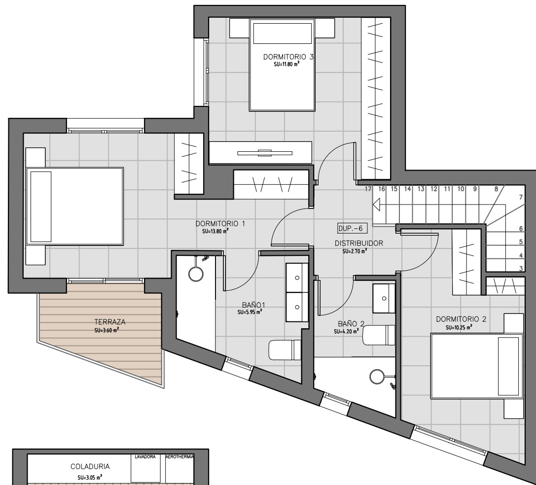
PLANTA PRIMERA
