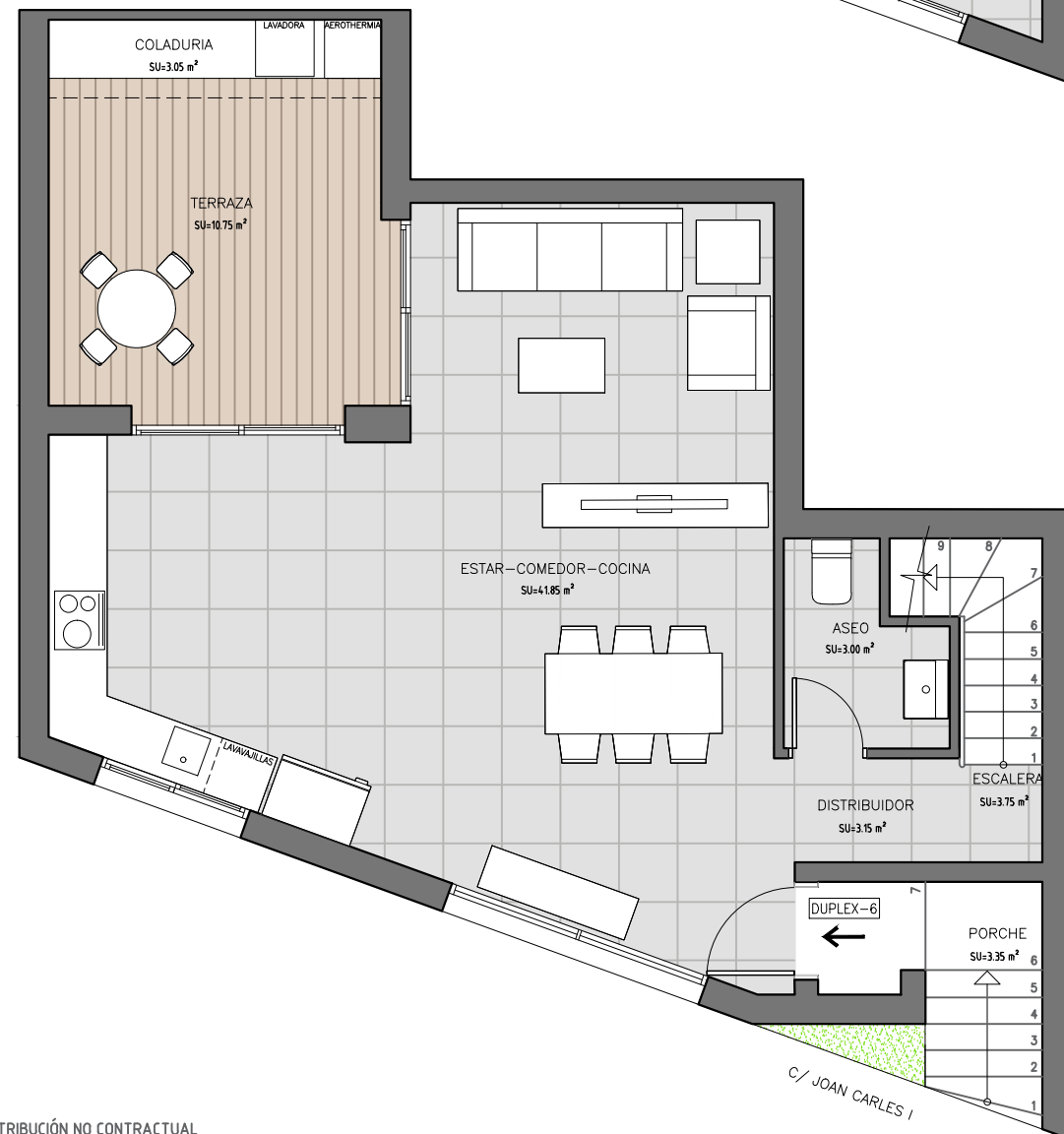
PLANTA BAJA
